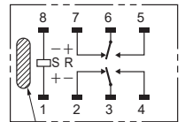
端子配置/内部连接图 (BOTTOM VIEW)
