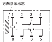
端子配置/内部连接图 (BOTTOM VIEW)
